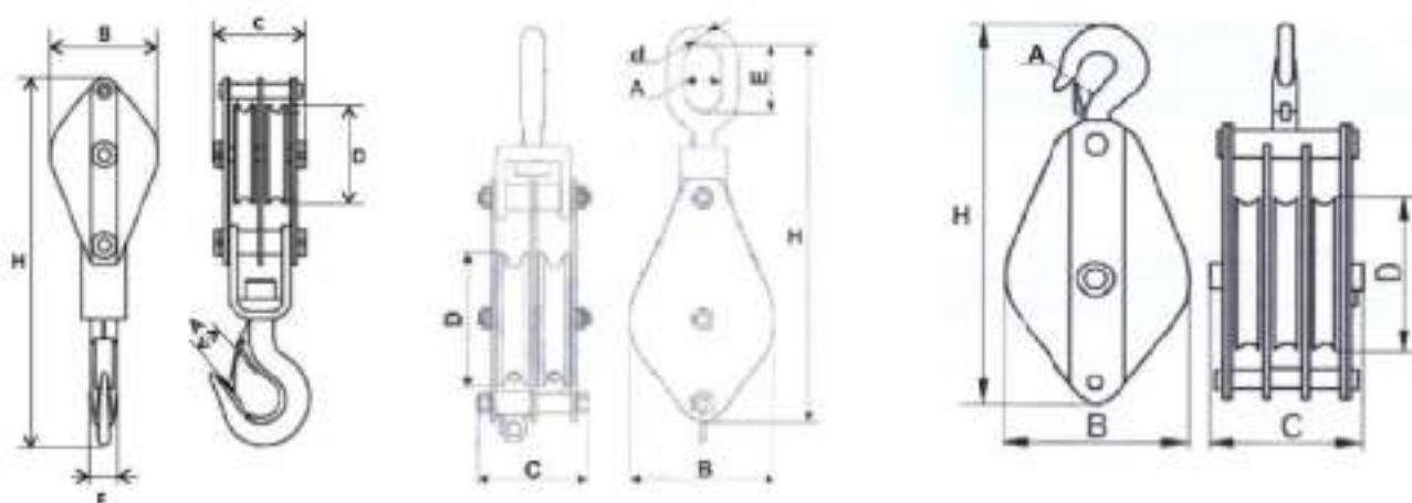
Рисунок 1. Размер блока
