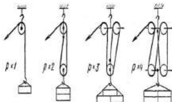
Рисунок 2. Применение блоков
