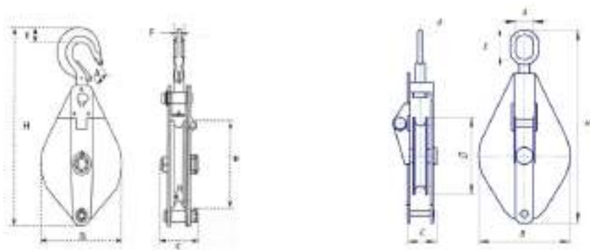
Рисунок 1. Размер блоков
