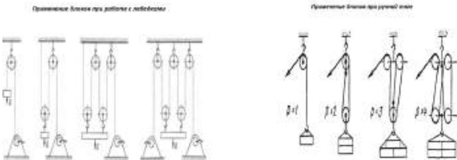
Рисунок 2. Применение блоков
