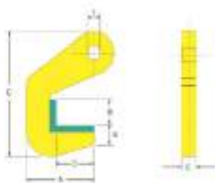
Рисунок 1. Размеры захвата
